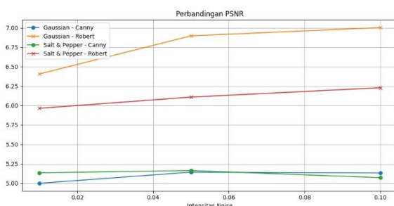
Gambar 5. Grafik PSNR
