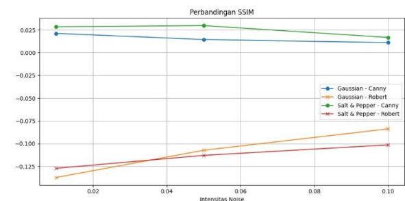
Gambar 7. Grafik SSIM
