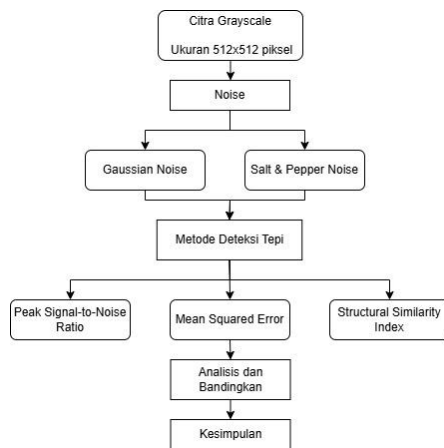
Gambar 2. Tahapan Penelitian
