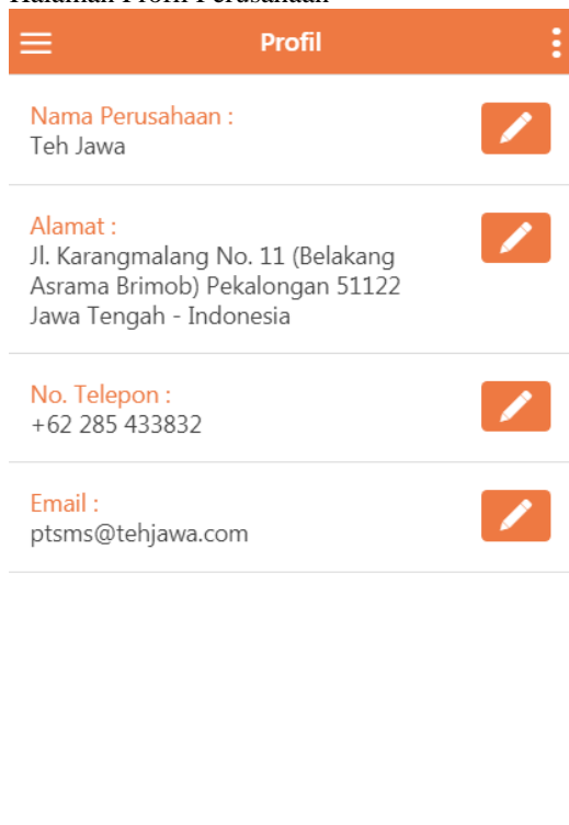
Gambar 4.7. Halaman Perusahaan
