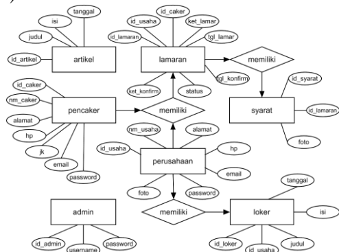
Gambar 3.10. Entity Relationship Diagram (ERD)
