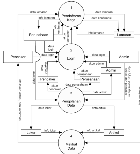
Gambar 3.7. DFD Level 0
