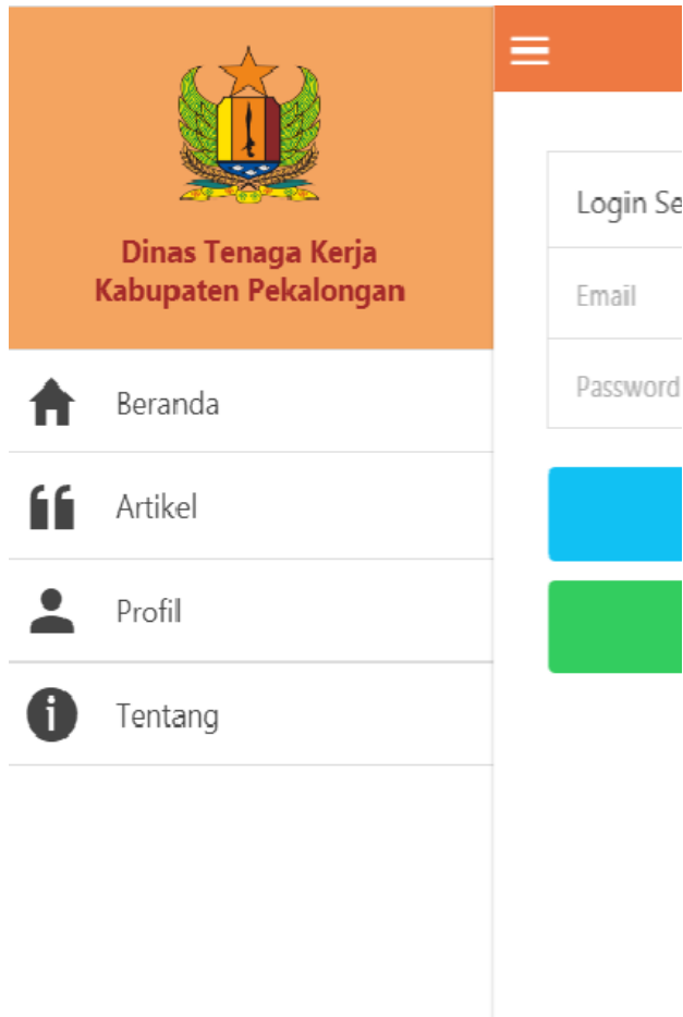
Gambar 4.2. Halaman Menu
