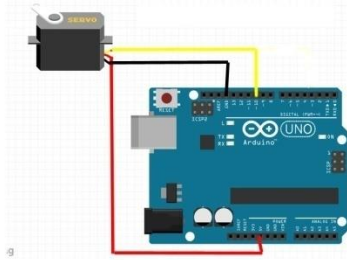
Gambar.4.11 Rangkaian penyambungan motor servo dengan arduino
